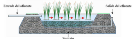
Figura 6. Humedal del flujo subsuperficial horizontal. Elaboración propia
