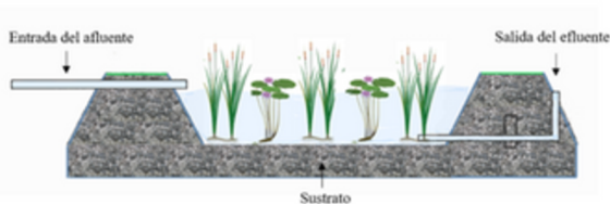
Figura 5. Humedal de flujo superficial. Elaboración propia
