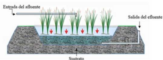
Figura 7. Humedal de flujo subsuperficial vertical. Elaboración propia
